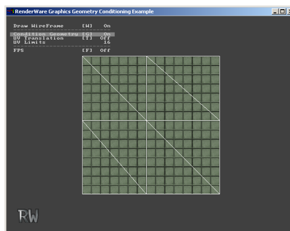
GCond Example
